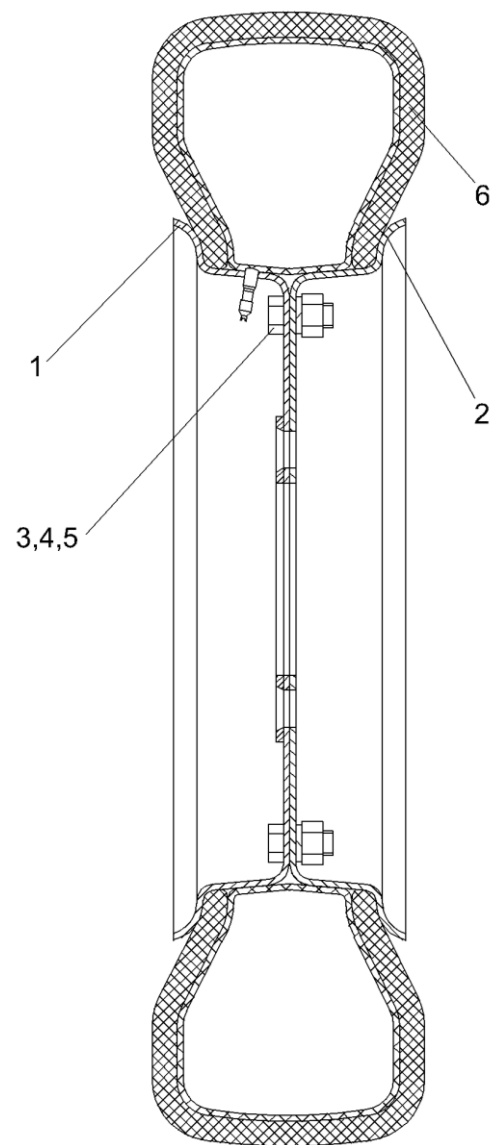
Рисунок 11 – Колесо 1925050
