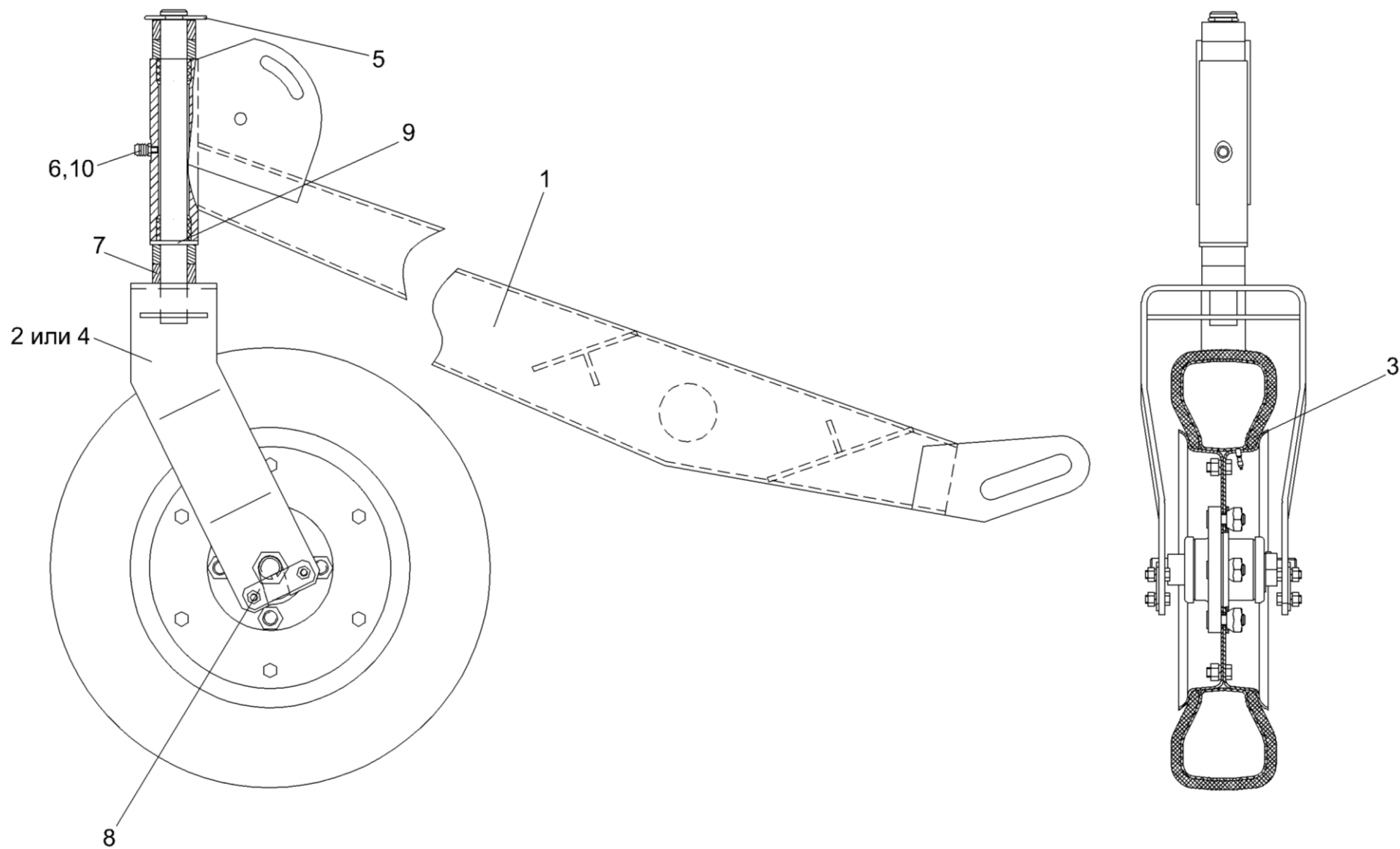
Рисунок 9 – Колесо КЗР 1925000
