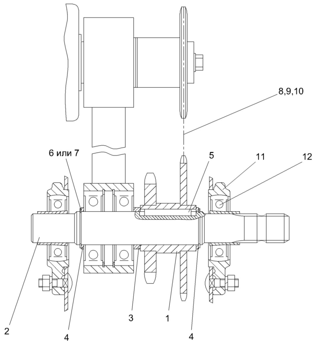
Рисунок 5 – Установка вала КЗК 1900601
